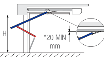
BTR - Porta basculante debordante a totale rientranza
