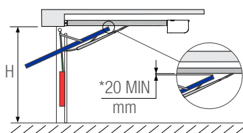
BPR - Porta basculante debordante a parziale rientranza (con ACG8201T)
